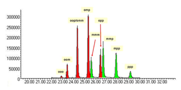
Abb. 2: SIM-Chromatogramm der Isomere des Trikresylphosphates
